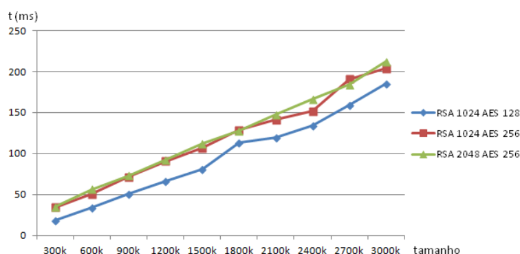
Figura 6. 2. Tempo de criptografia dos arquivos
