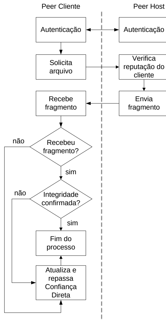
Figura 5.7. Processo de interação entre peers.
