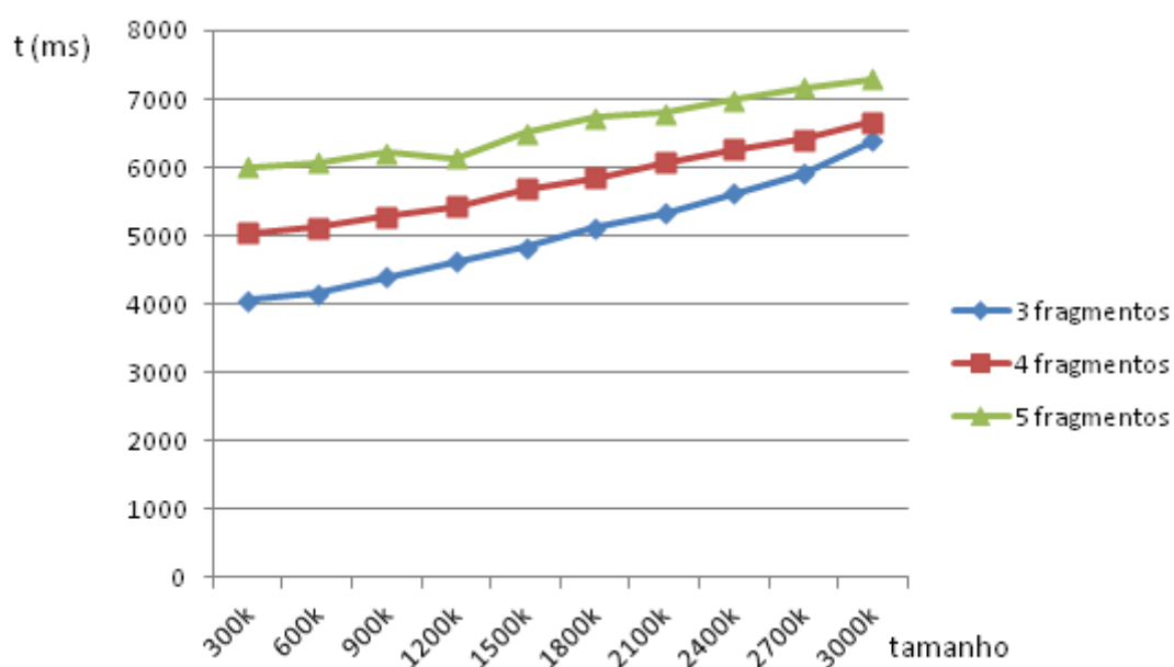
Figura 6. 6. Tempos de recuperação em rede local com RSA 2048 AES 256.
