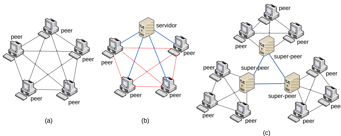
Figura 2.3. Topologias P2P. (a) Pura. (b) Híbrida. (c) Super-peer.
