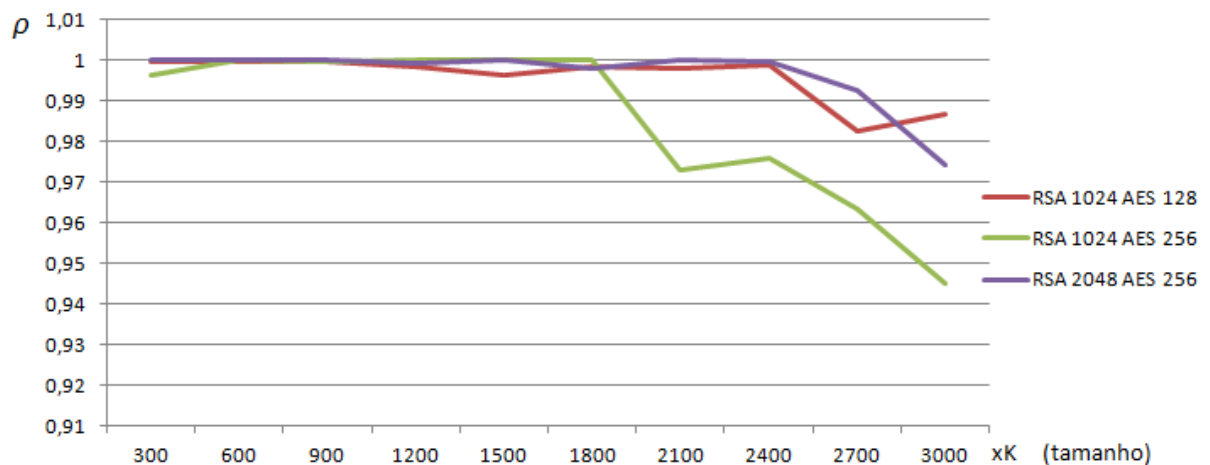
Figura 6. 7. Correlação entre fragmentação do arquivo e tempo de recuperação.
