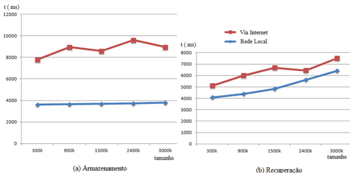
Figura 6. 9. Armazenamento e recuperação em rede local e via Internet.
