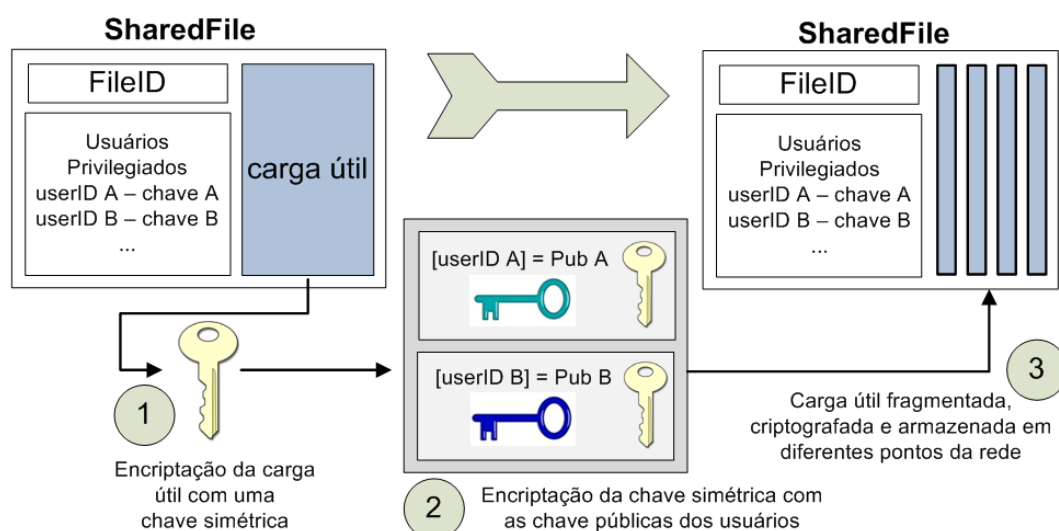
Figura 5.1. Esquema de criptografia do SharedFile .
