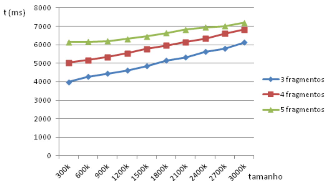
Figura 6. 4. Tempos de recuperação em rede local com RSA 1024 AES 128.
