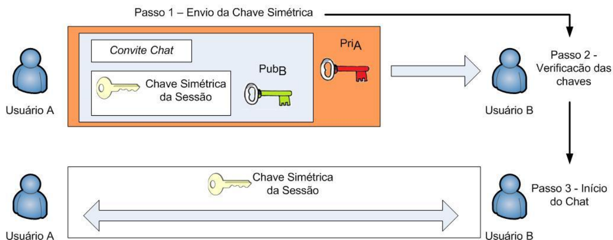
Figura 5.4 Esquema de Comunicação Segura (Chat).
