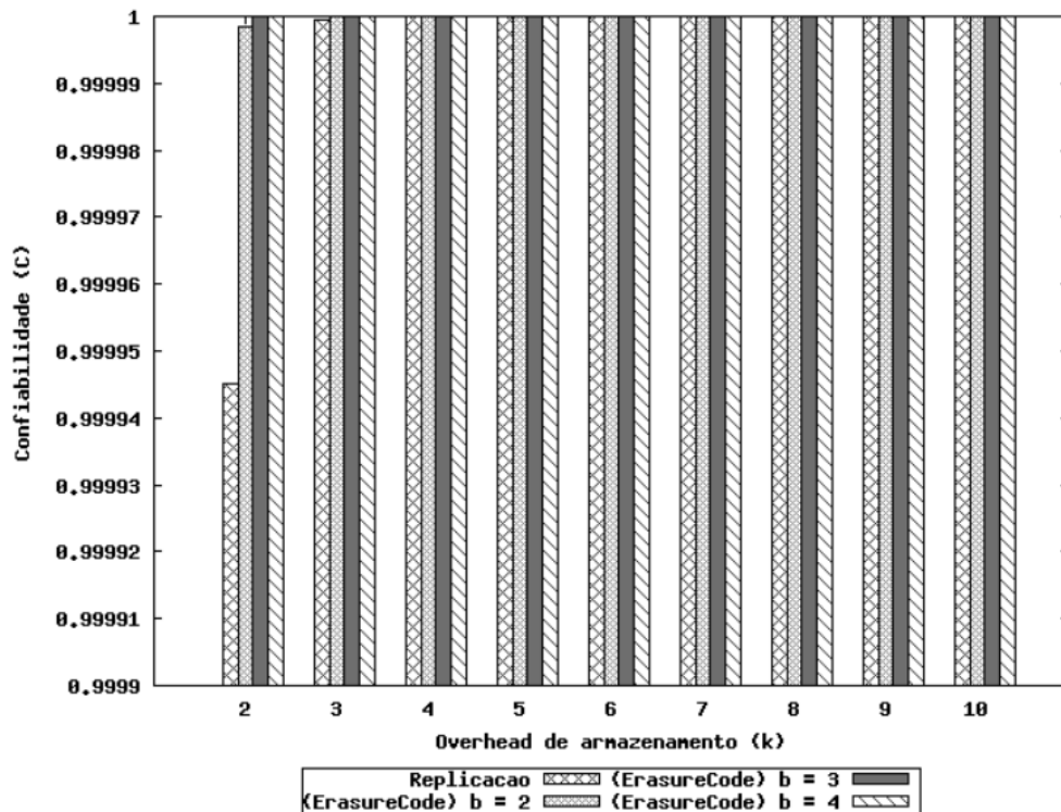
Figura 2.4. Comparação entre a confiabilidade obtida usando Replicação e Erasure codes diante de ocorrência de falhas de disco ( f=0,0074 ) [Oliveira 2007.]
