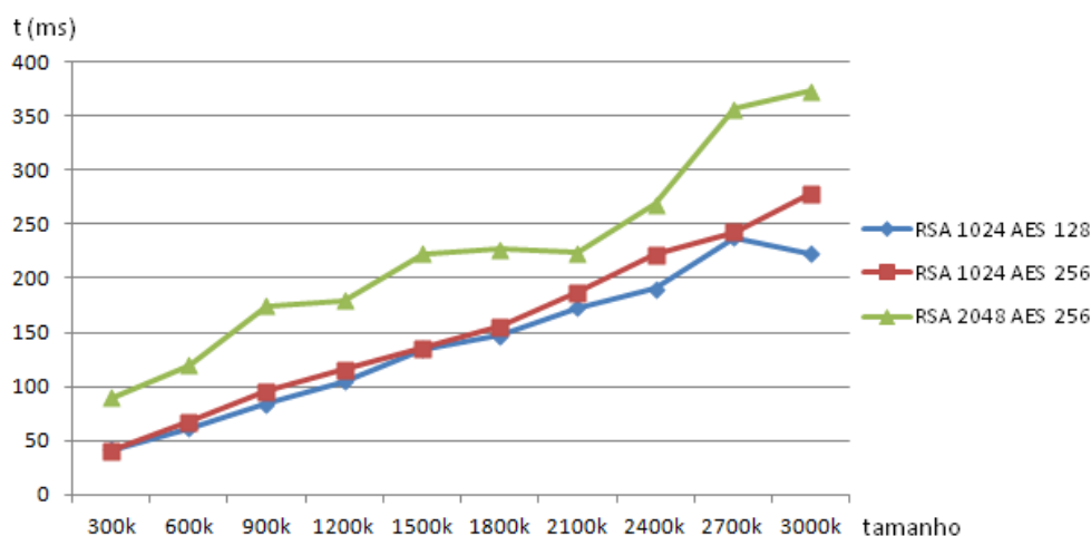
Figura 6. 3 Tempo de descryptografia dos arquivos
