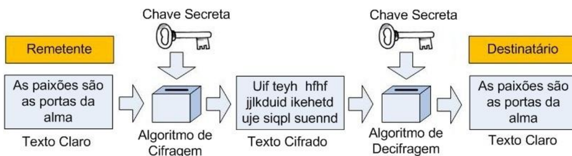
Figura 2.6. Esquema de Criptografia por Chave Simétrica.
