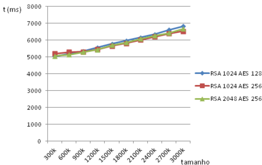
Figura 6. 8. Tempo de recuperação de arquivos (4 fragmentos).
