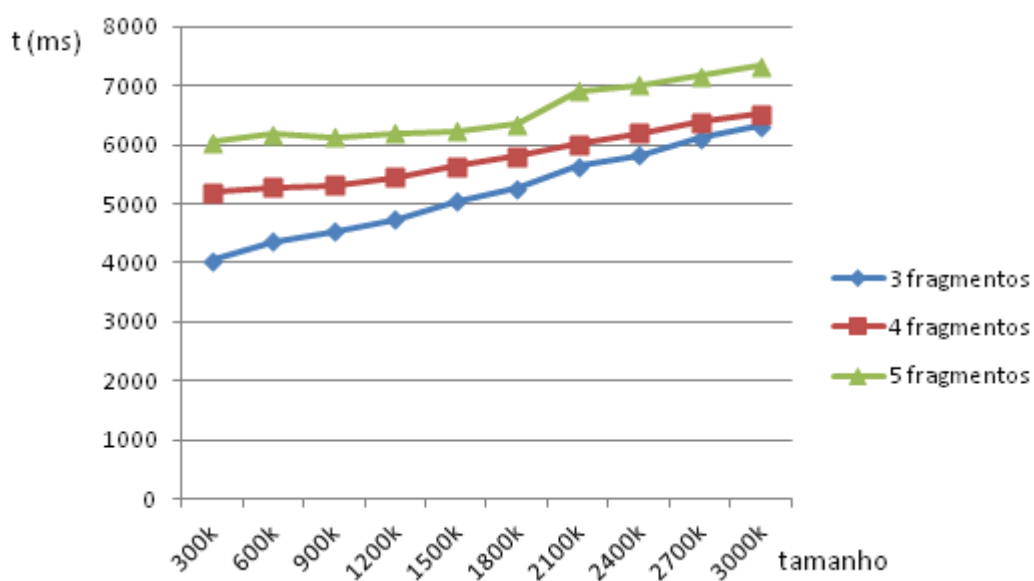
Figura 6. 5. Tempos de recuperação em rede local com RSA 1024 AES 256.
