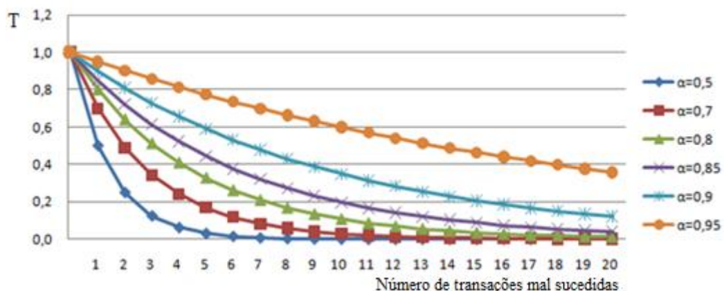
Figura 5.5 Variação da Reputação em função do número de interações comprometidas.
