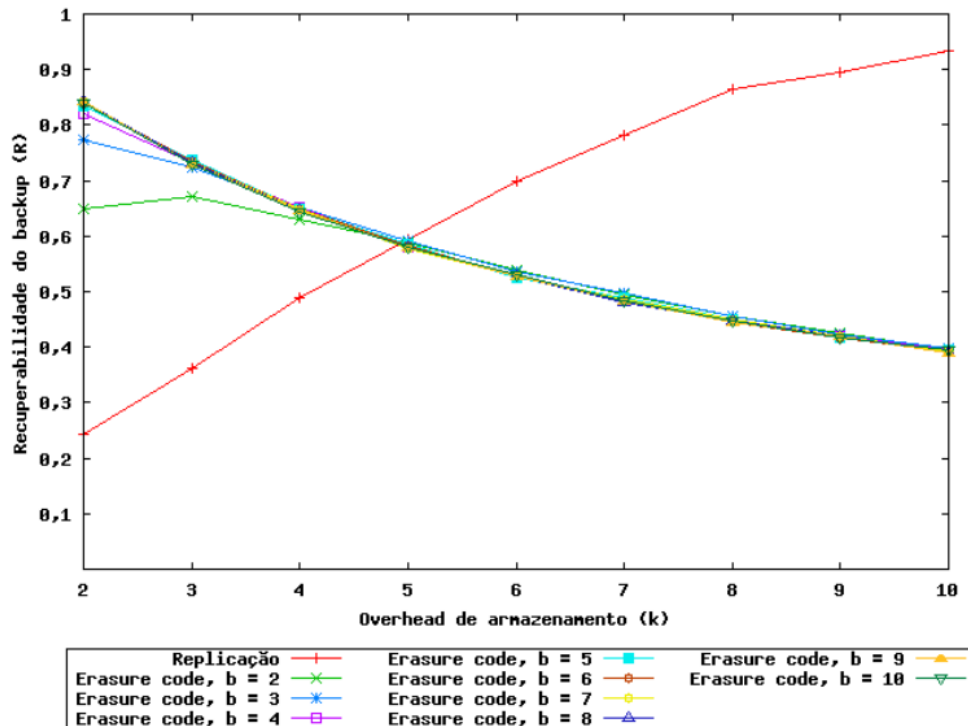
Figura 2.5. Replicação vs. Erasure Code [Oliveira 2007].
