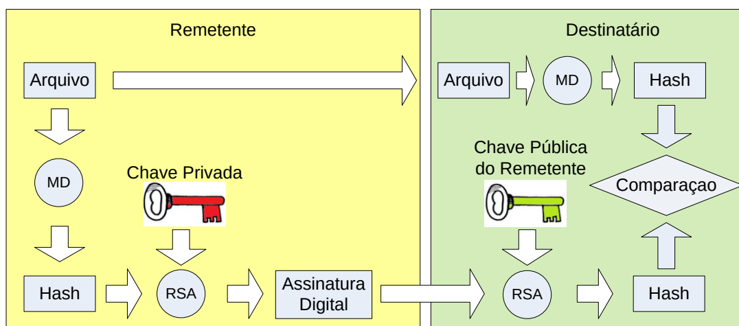
Figura 2. 8. Esquema de Assinatura Digital.
