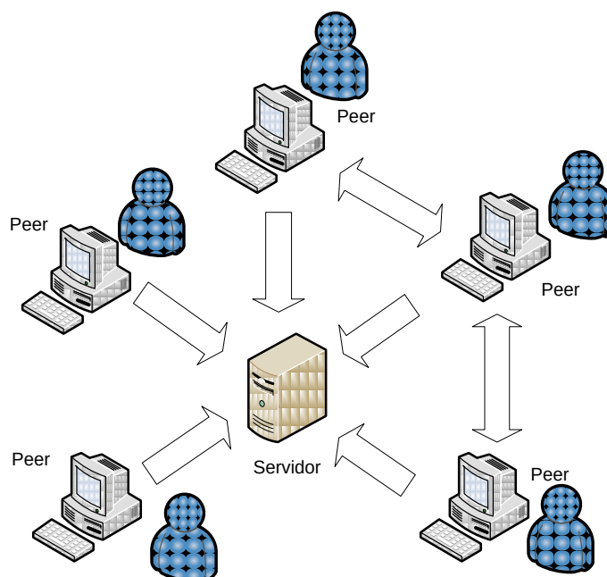
Figura 4.2 Macro-arquitetura da Rede de Confiança.
