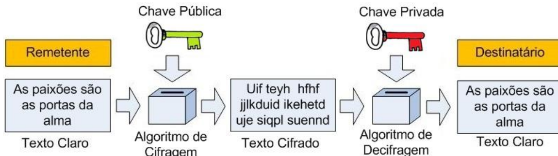
Figura 2.7. Esquema de Criptografia por Chave Assimétrica.
