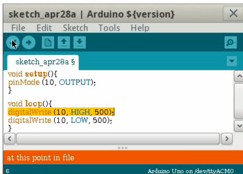
Figura 15: Passagem de parâmetros errada
