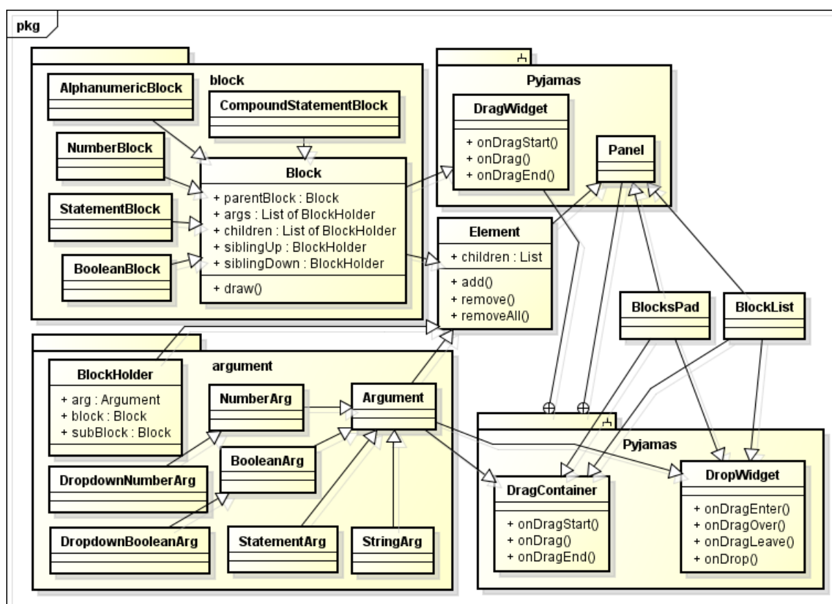
Figura 49: Diagrama de Classes Resumido do DuinoBlocks
