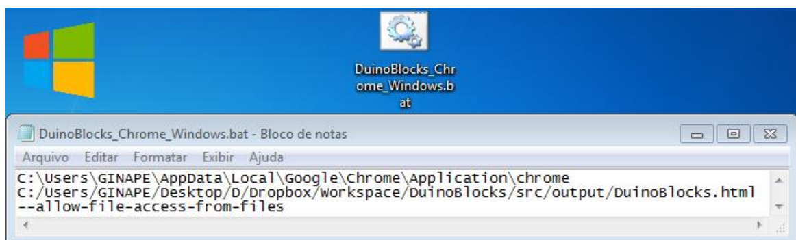
Figura 51: Código para executar o DuinoBlocks no modo off-line com o Chrome no Windows
