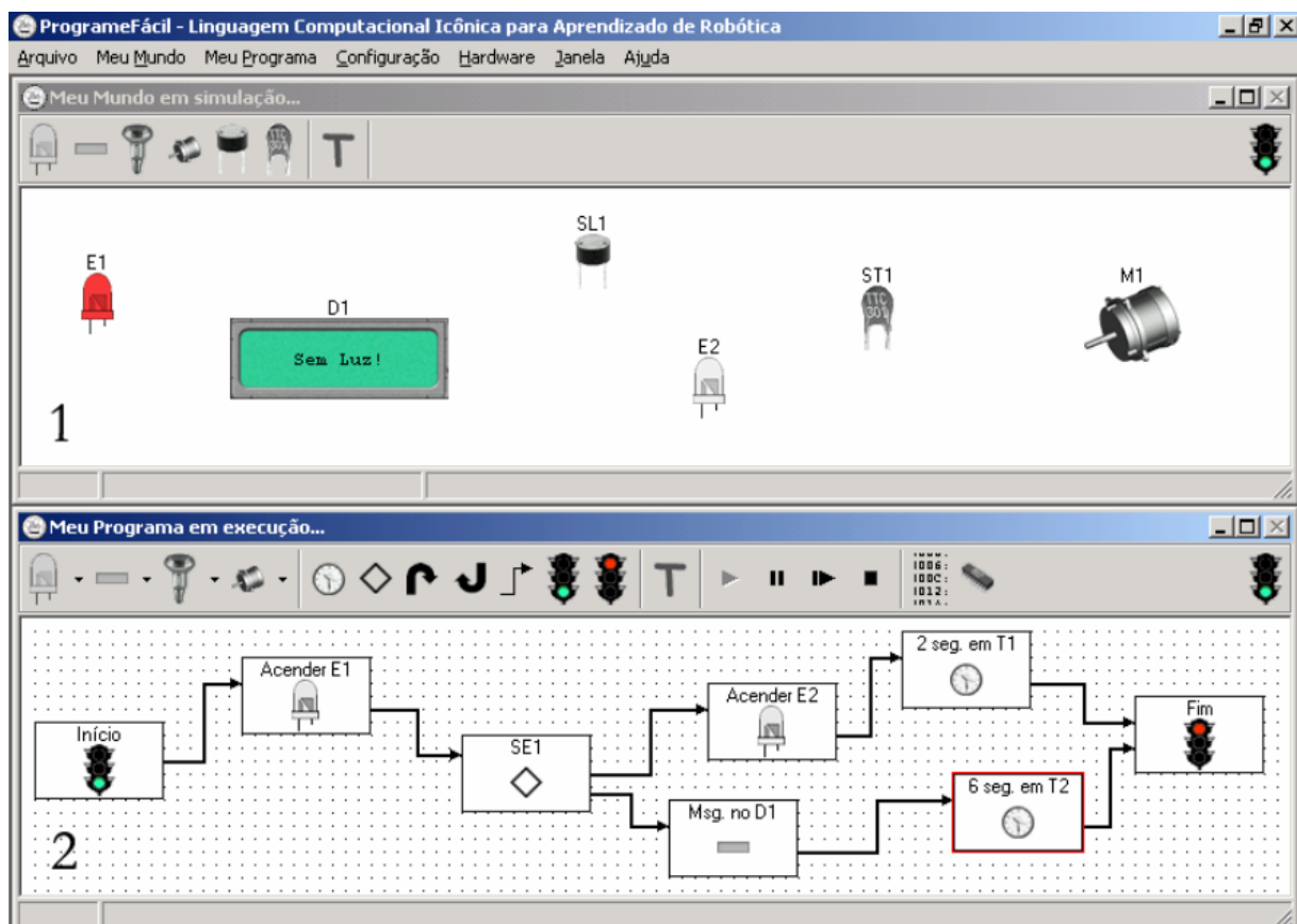
Figura 6: ProgameFácil – Linguagem Computacional Icônica para Aprendizado de Robótica
