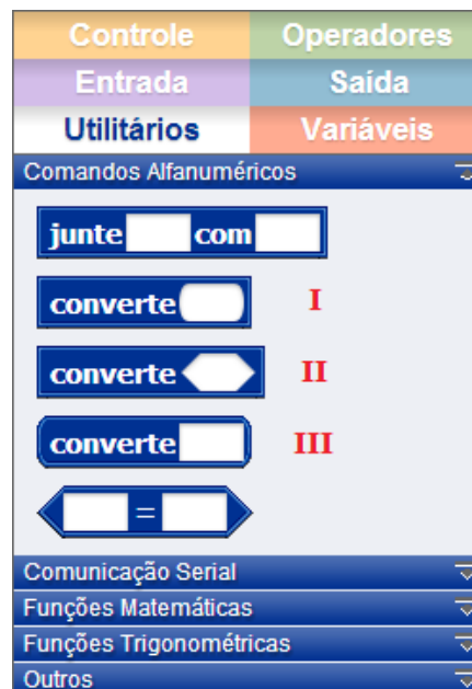
Figura 27: Blocos “converte” da subcategoria “Comandos Alfanuméricos” em “Utilitários”
