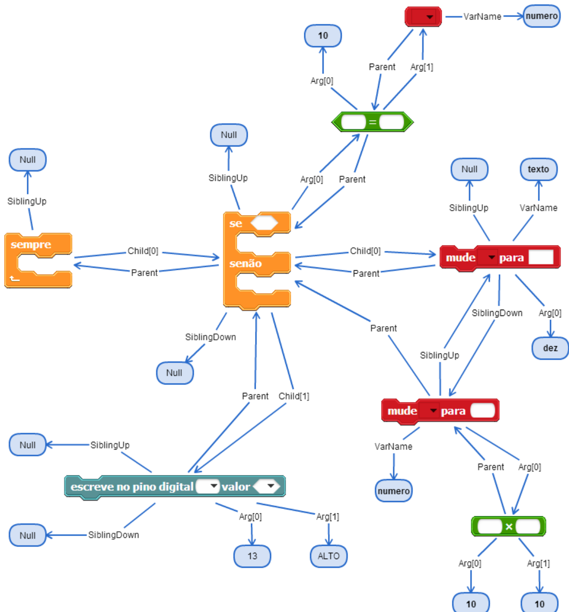
Figura 48: Estrutura lógica do exemplo de pilha da Figura 47
