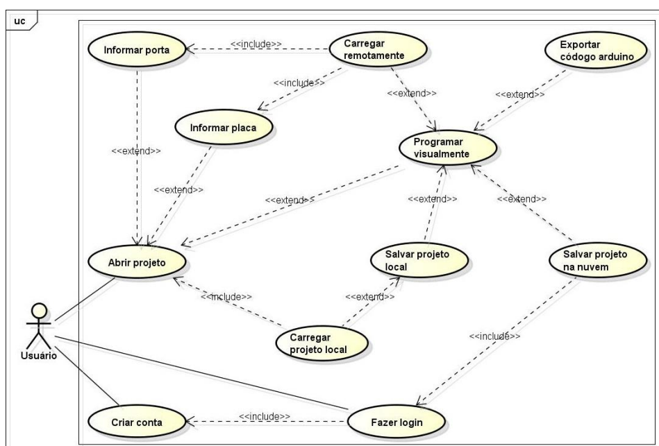
Figura 17: Diagrama de Caso de Uso.
