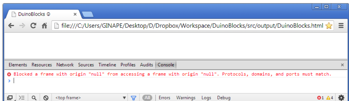
Figura 50: Erro ao executar o DuinoBlocks com o Chrome
