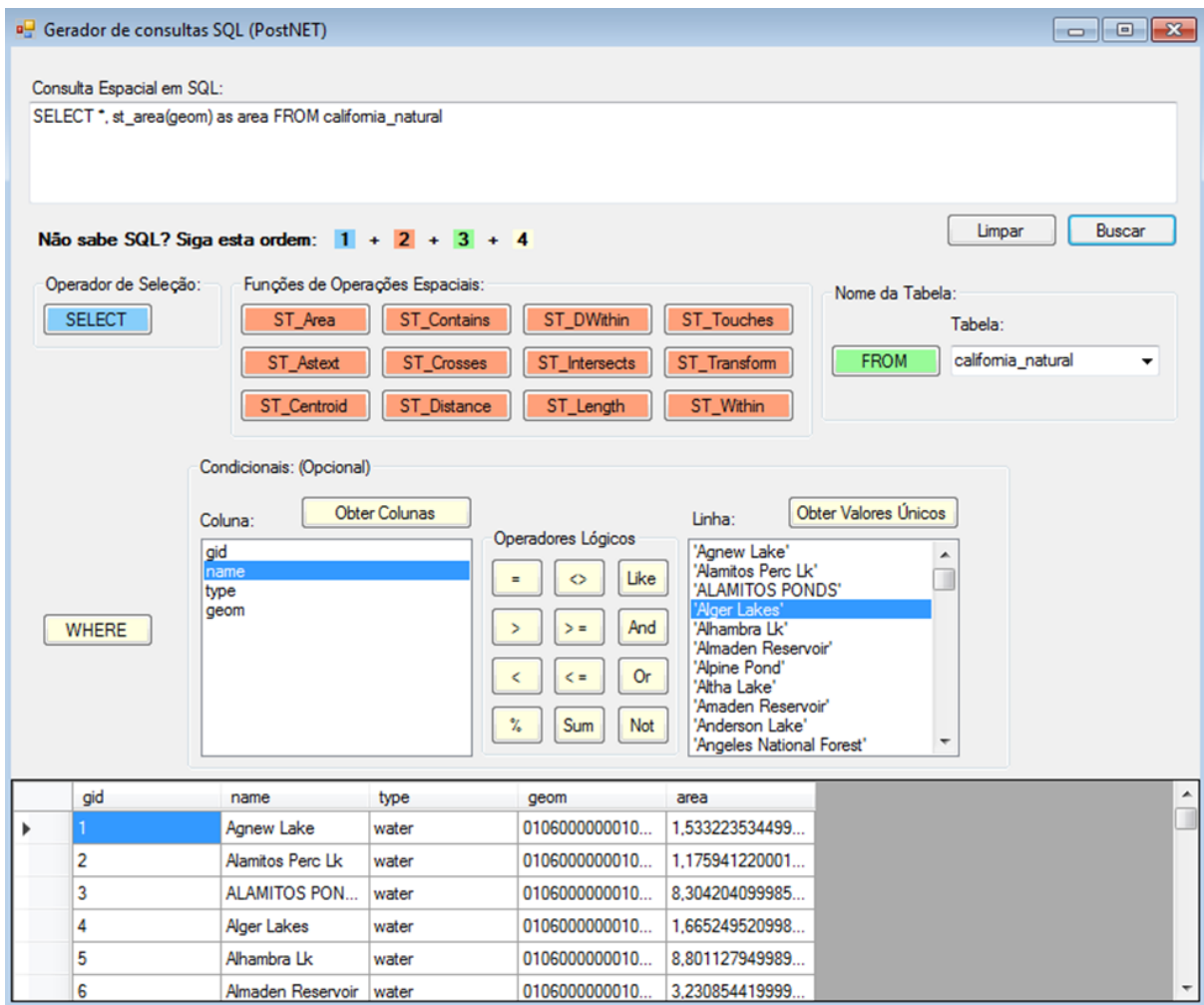
Figura A.1: Interface gráfica do Gerador de Consultas SQL (PostGIS)
