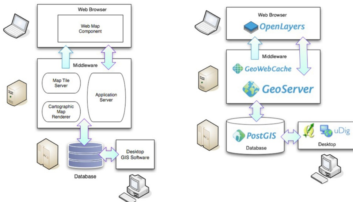
Figura 8.8: : Estrutura de código aberto que foi utilizada no trabalho e a representação da interface usuário/servidor. Autor: Carlos Cesar Gomes São Braz - IME(RJ)
