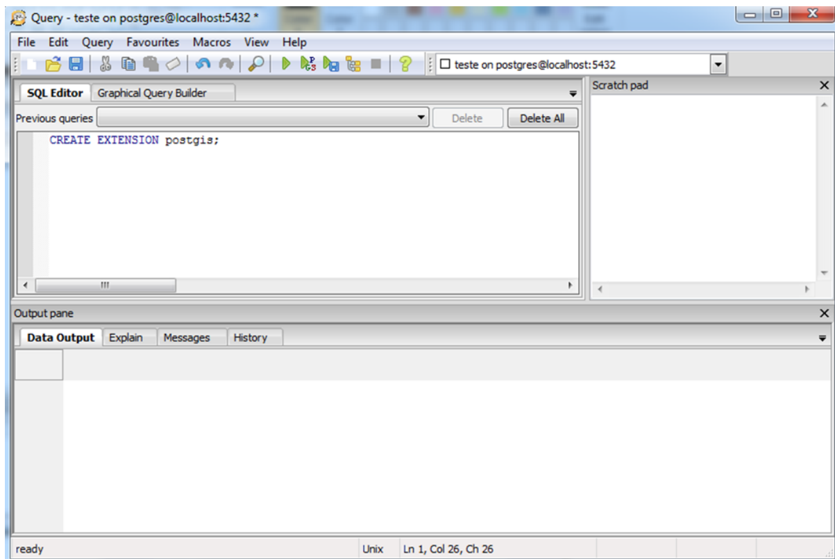
Figura 8.4: Através da consulta ” create extension postgis ” o banco recém-criado já poderá utilizar as funcionalidades espaciais.
