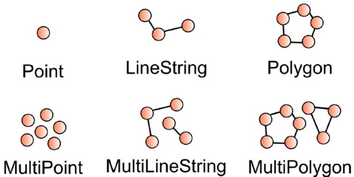
Figura 6.17: Tipos geométricos básicos suportados pela SFS-SQL. [75]
