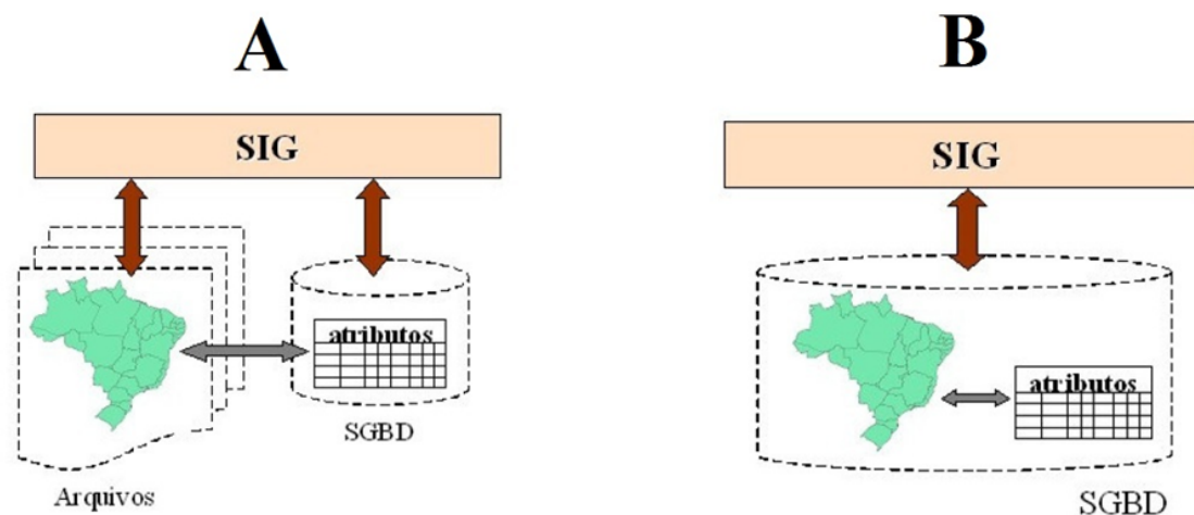
Figura 6.16: (A) Arquitetura Dual; (B) Arquitetura Integrada. CASANOVA et al. (2005)
