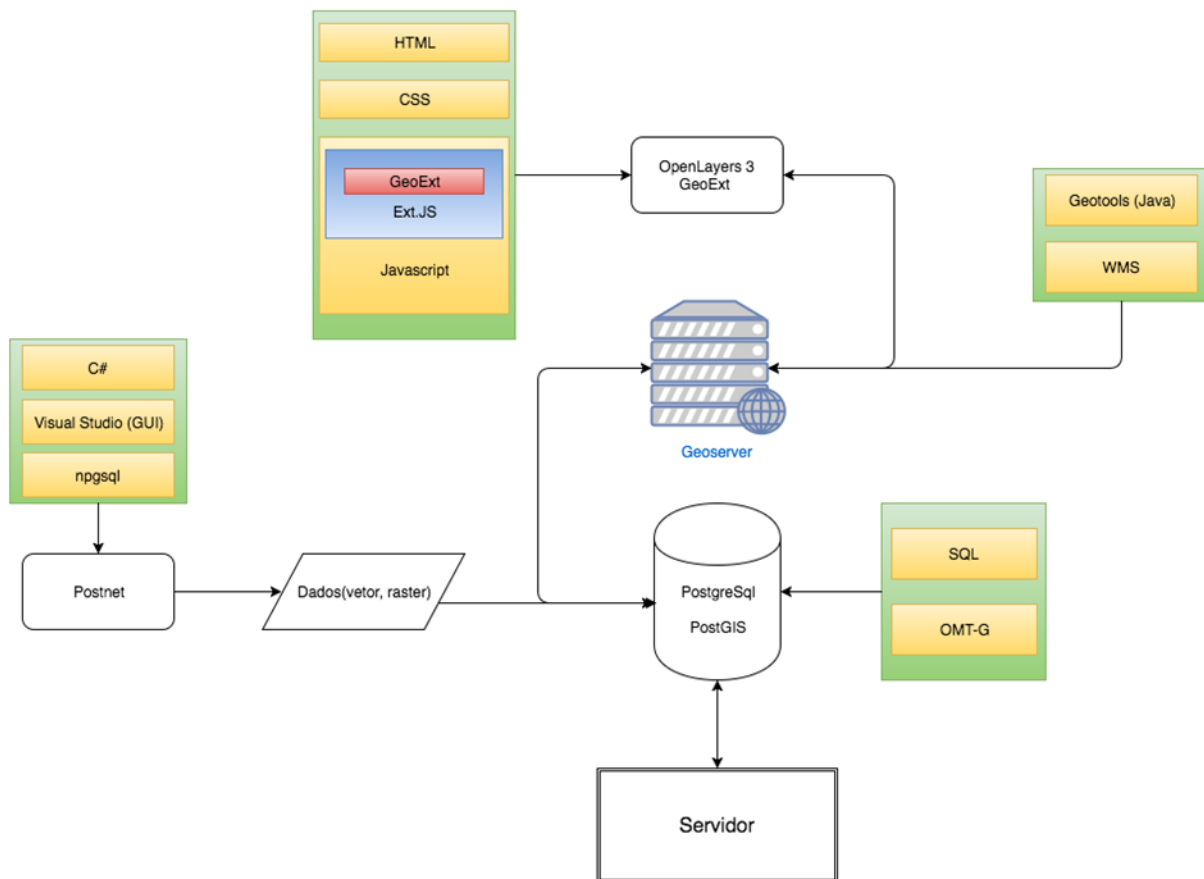
Figura 8.9: Diagrama com as ferramentas de análise, linguagens, recursos, suas conexões, camadas de abstração e tecnologias envolvidas.
