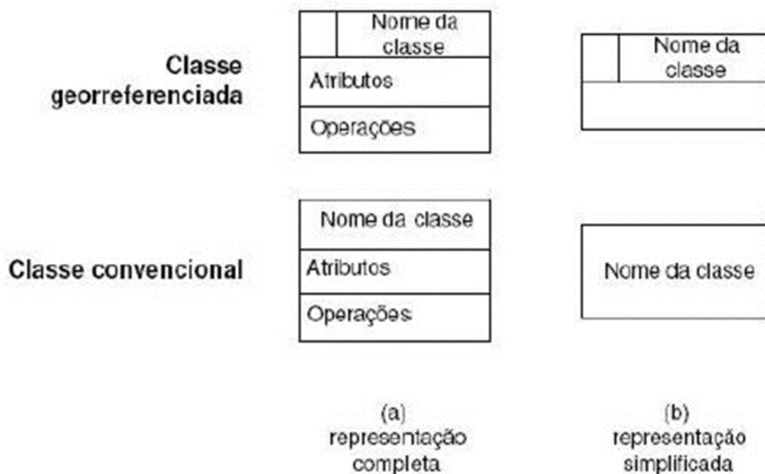
Figura 6.3: Classes georreferenciadas e convencionais no OMT-G.[63]
