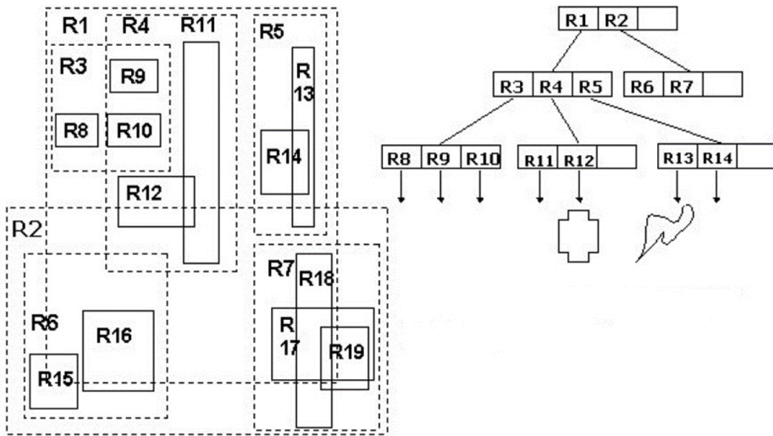
Figura 6.18: Árvore-R. Modificado de Queiroz & Ferreira (2006)
