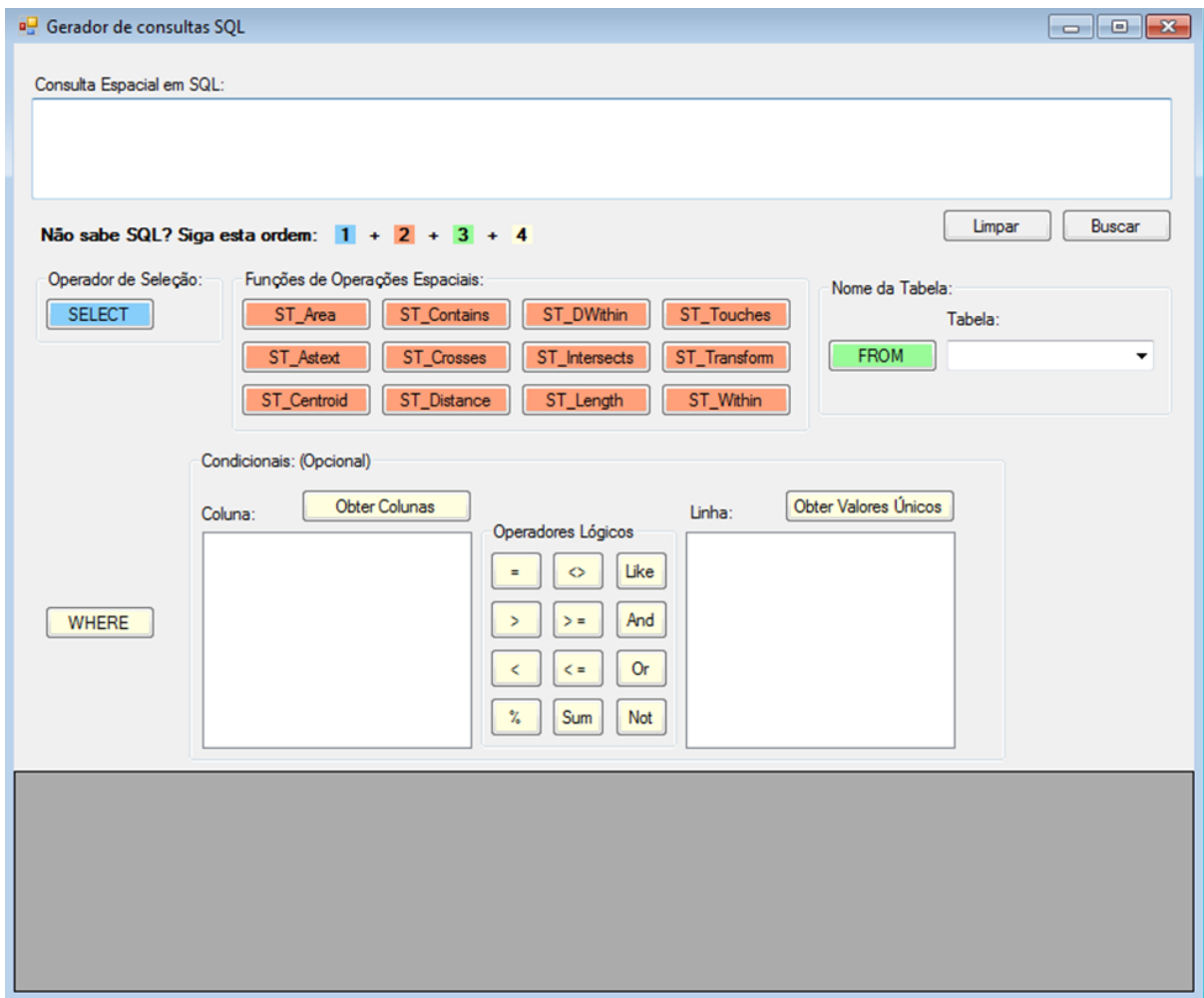
Figura 8.13: Módulo PostNET ou "Gerenciador de Consultas SQL".
