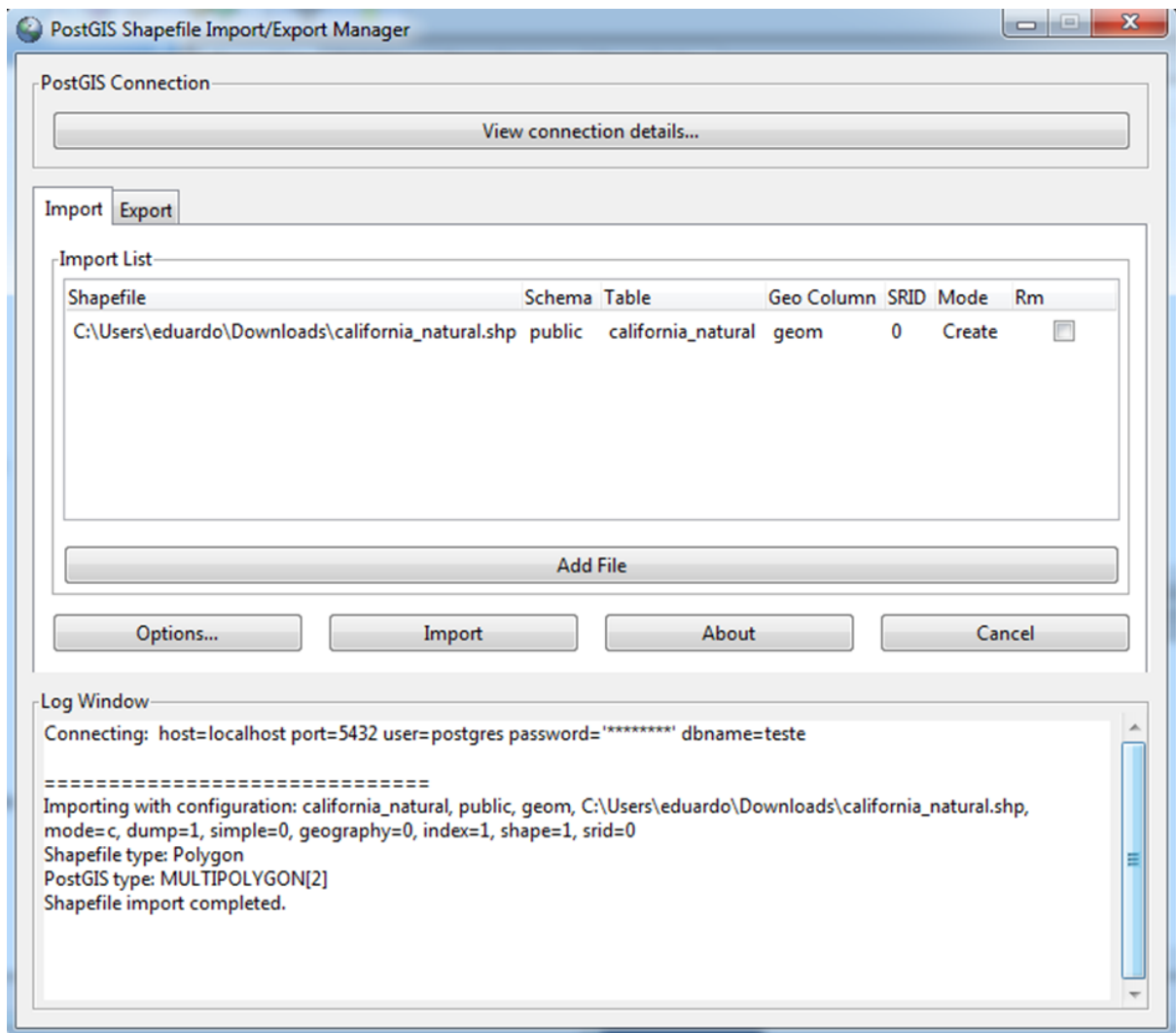
Figura 8.6: Interface gráfica do Shapefile and DBF Loader 2.1.
