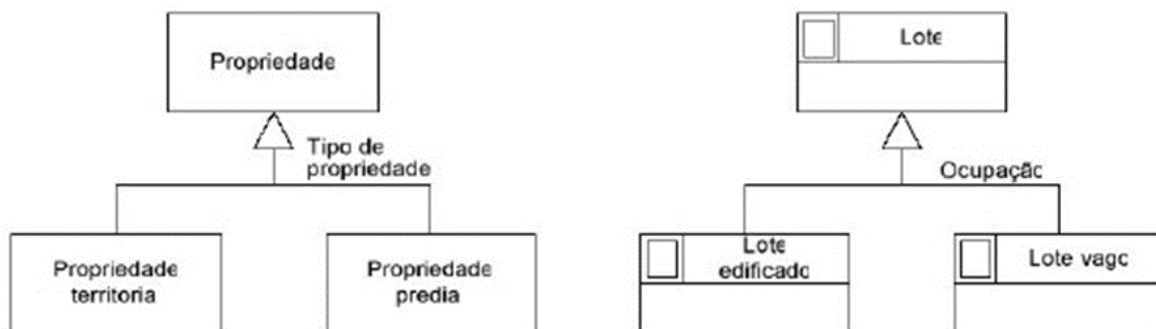
Figura 6.9: Generalização/Especialização. [63]
