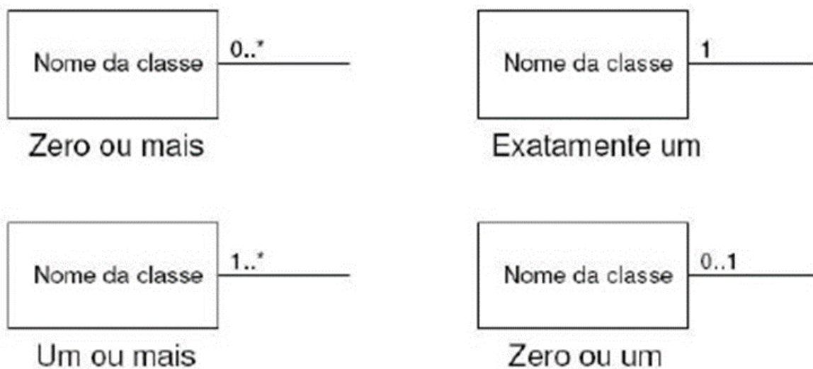
Figura 6.7: Cardinalidade. [63]
