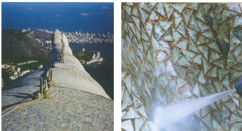
Figura 37 (esquerda) – Instalação da proteção catódica. Figura 38 (direita) – Limpeza e recuperação do mosaico. Fonte: FUNDAÇÃO ROBERTO MARINHO, 2005.
