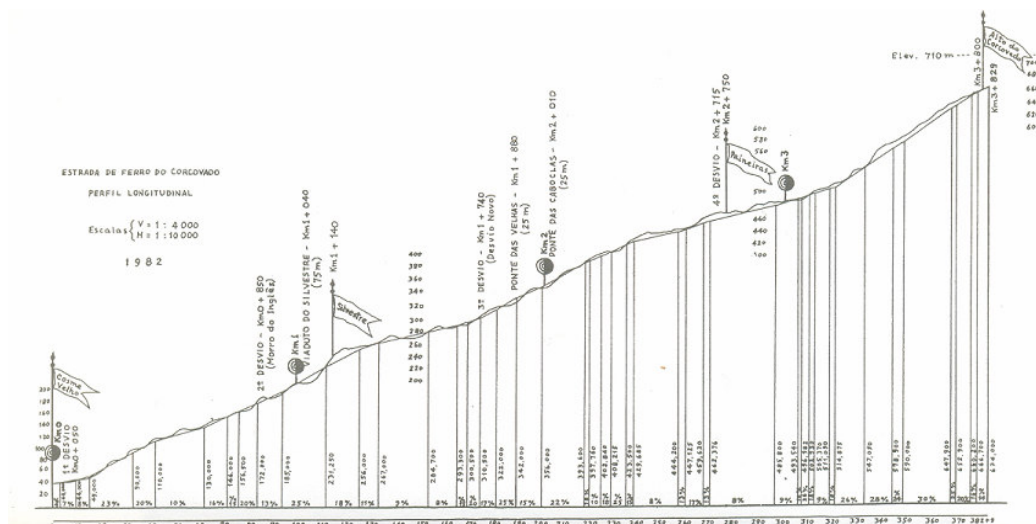
Figura 11 – Perfil longitudinal da Estrada de Ferro do Corcovado (1904). Fonte: SEMENOVITCH, 1997.
