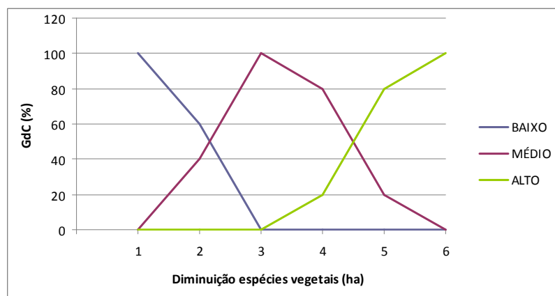
Figura 2.5 : Conjuntos Fuzzy variável entrada “Diminuição espécies vegetais uso herbicidas”
