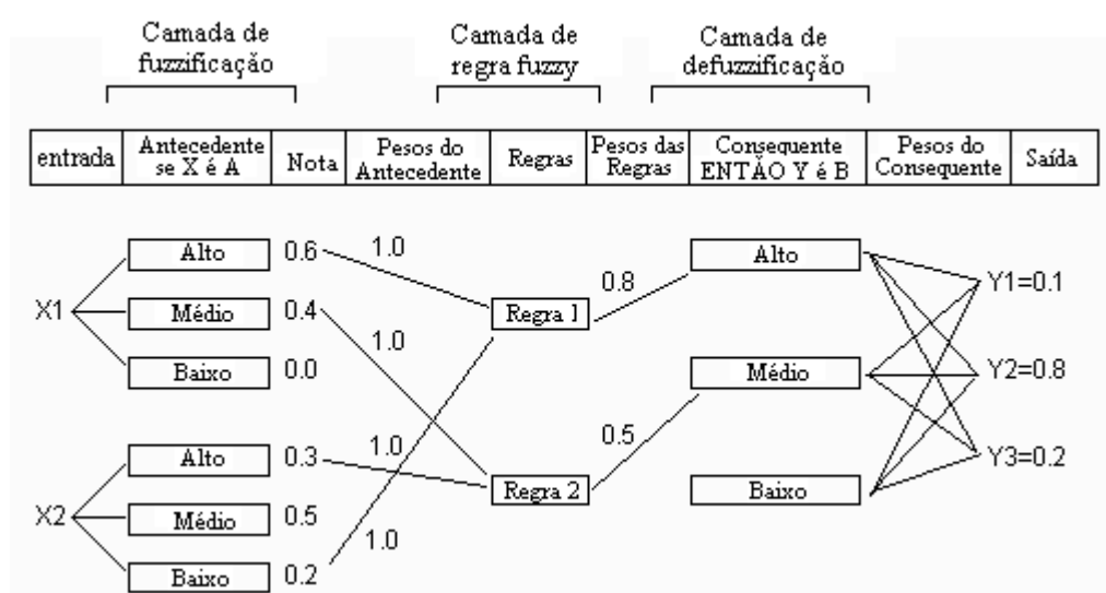
Figura 3.17: Exemplo de um sistema Neuro-Fuzzy
