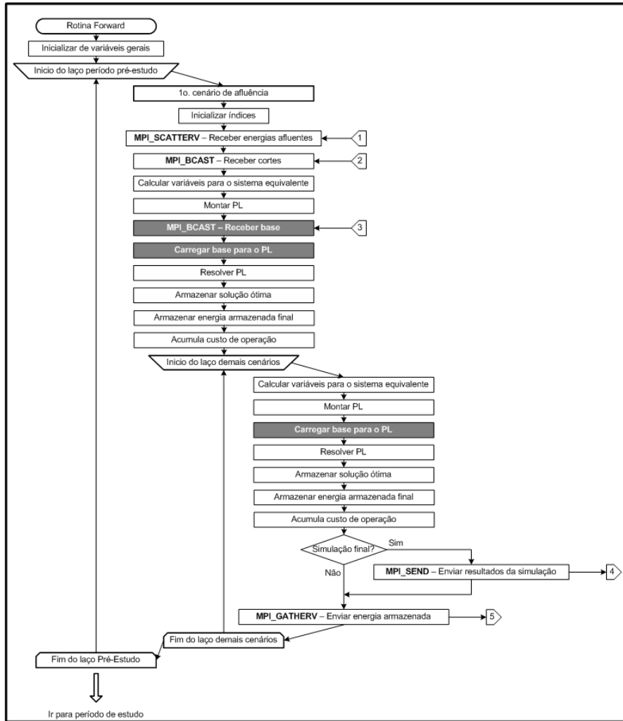
Figura 118 - Fluxograma da Rotina Forward com Envio de Base (Demais Processadores)
