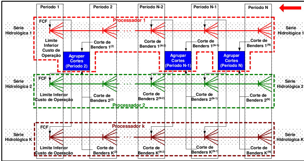
Figura 38 – Distribuição dos Cortes de Benders no Processo Backward
