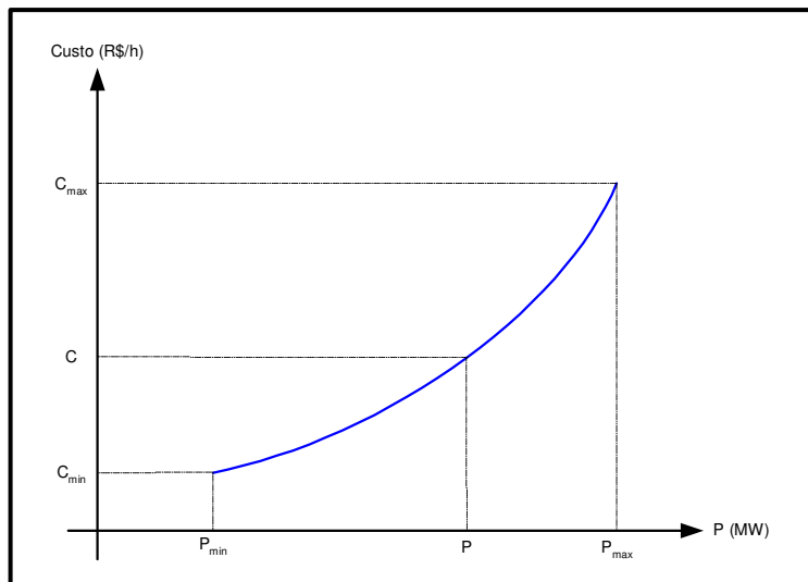
Figura 4 – Custo de Produção Típico de Uma Usina Térmica
