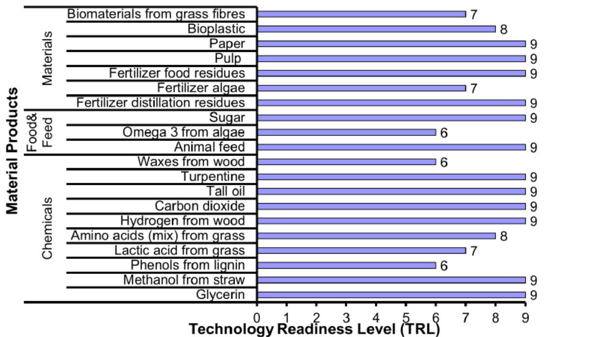
Figura 26: TRL para produtos
