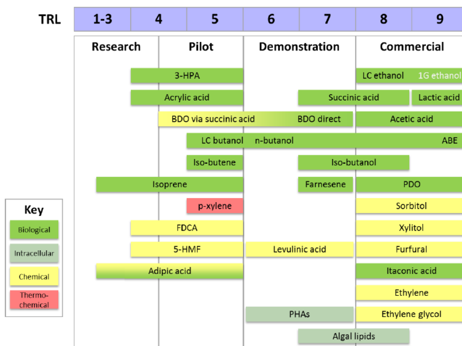
Figura 8: Estado de Comercialização de 25 produtos selecionados da plataforma de açúcar. Fonte: (E4TECH et al. , 2015)
