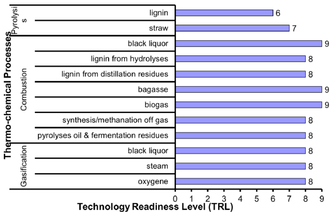
Figura 27: TRL para processos termoquímicos
