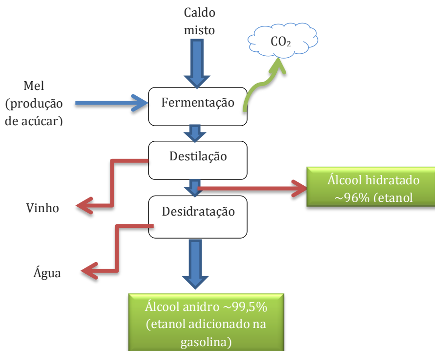
Figura 22: Produção do etanol
