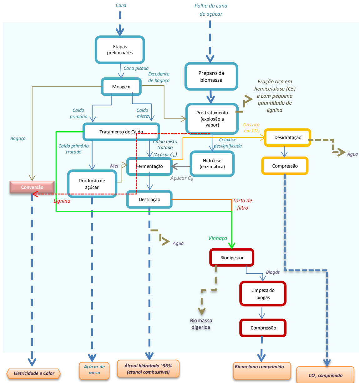
Figura 14: Fluxograma da Biorrefinaria hipotética V1
