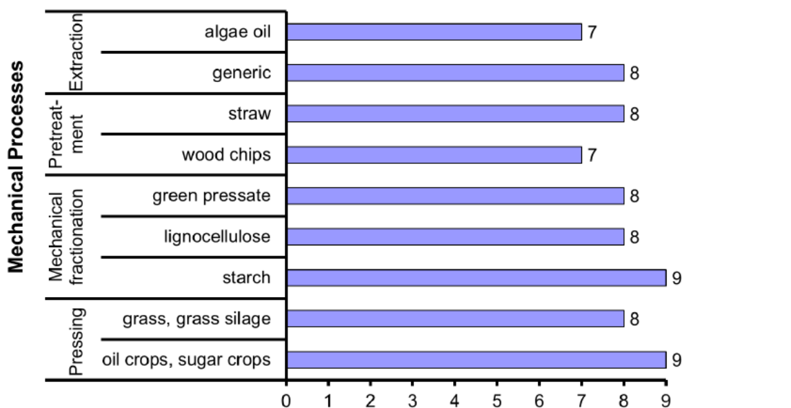
Figura 30: TRL de processos mecânicos I
