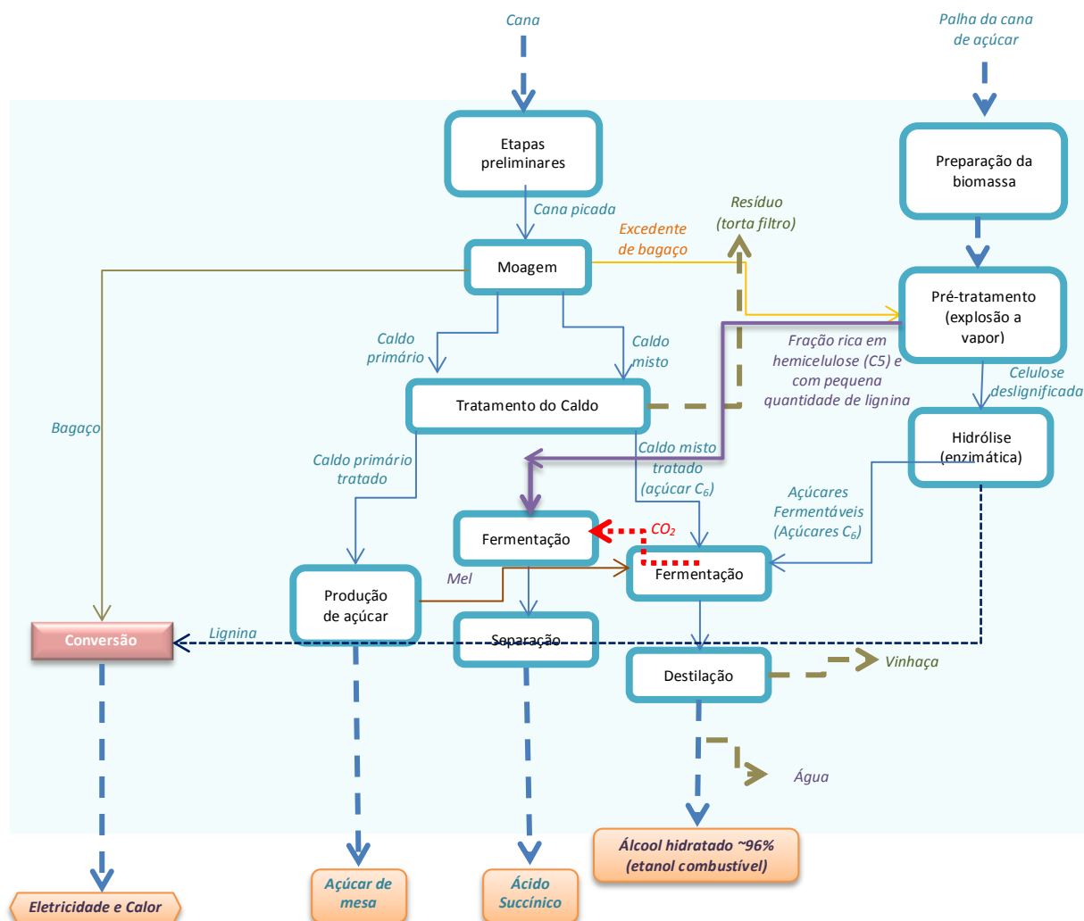
Figura 13: Fluxograma da Biorrefinaria D1
