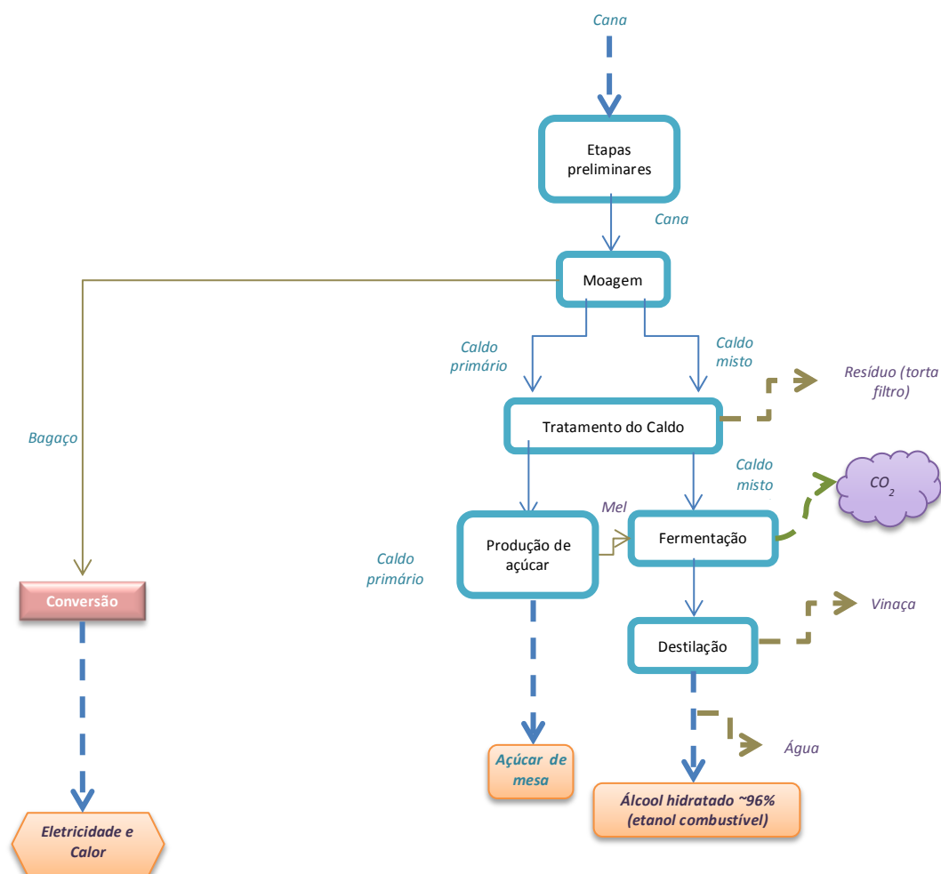
Figura 10: Fluxograma da Biorrefinaria A1
