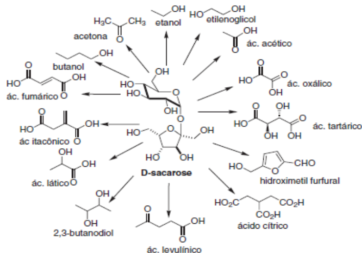
Figura 4: Alguns produtos químicos com baixas massas moleculares obtidos a partir da sacarose (ANTUNES et al. , 2010)
