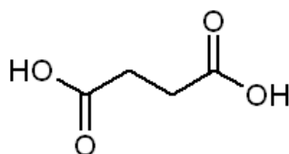
Figura 7: Estrutura química do ácido butanodióico
