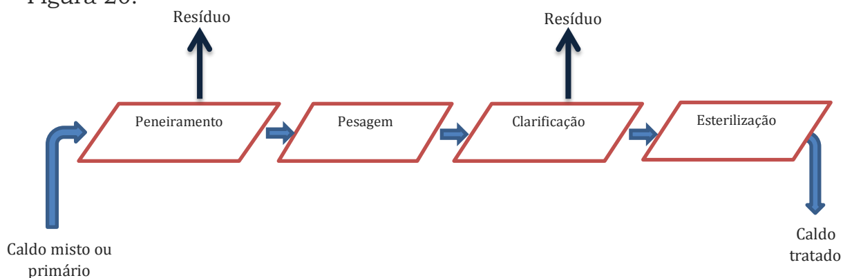
Figura 20: Etapa de tratamento do caldo
