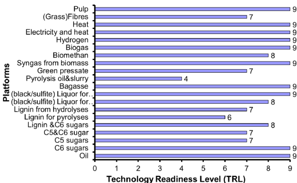
Figura 23: TRL para plataformas
