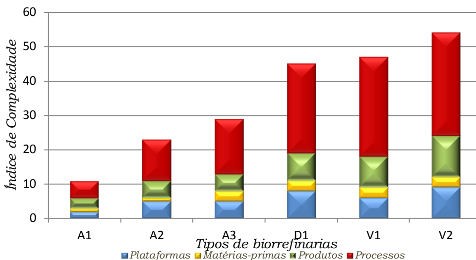
Figura 17: Gráfico complexidade das biorrefinarias estudadas
