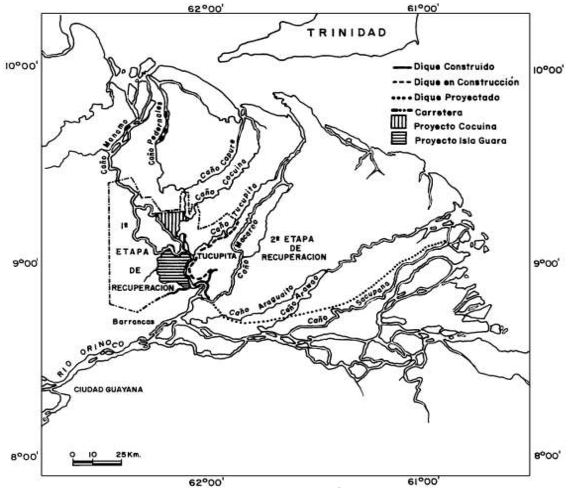
Figura 5 – Projeto das obras no delta do rio Orinoco
